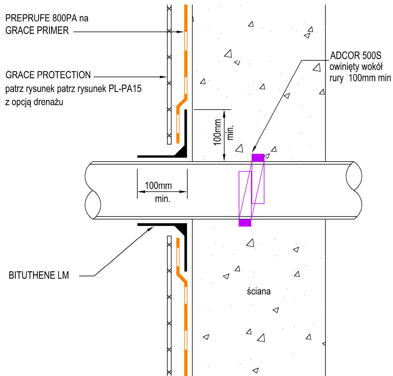
PRZEJŚCIE RURY PRZEZ ŚCIANĘ RZUT/ PRZEKRÓJ
